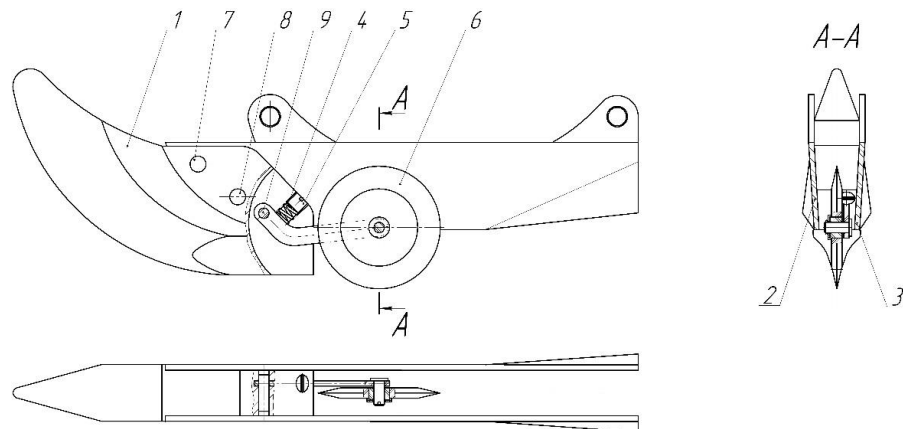
Рис. 2. Удосконалений сошник
