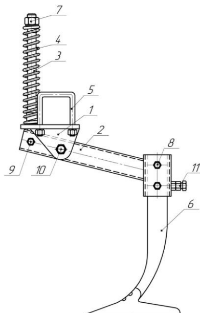
Рис.1. Експериментальна секція парового культиватора.
