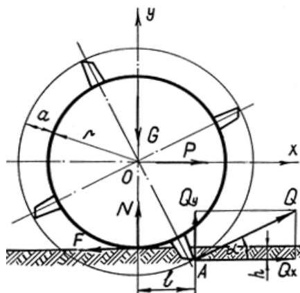
Рис. 1. Расчетная схема посевного колеса.
