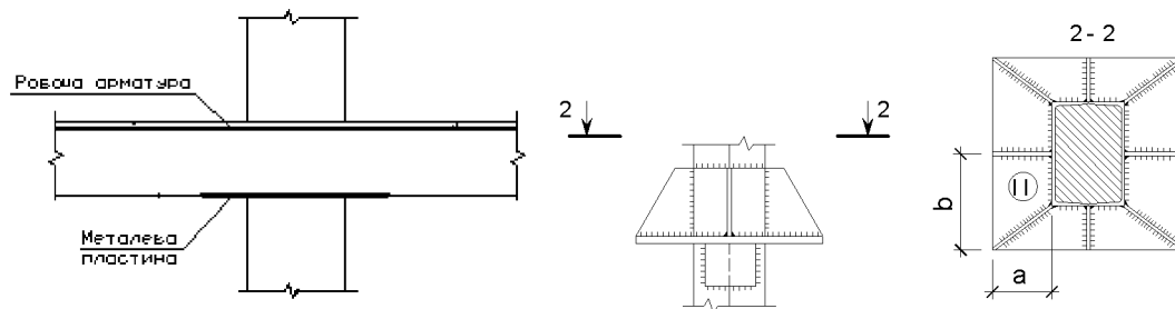
Рисунок 1 - Розрахункова схема вузла сталезалізобетонної колони із залізобетонним монолітним переkritтям та конструкція опорної плити вузла
