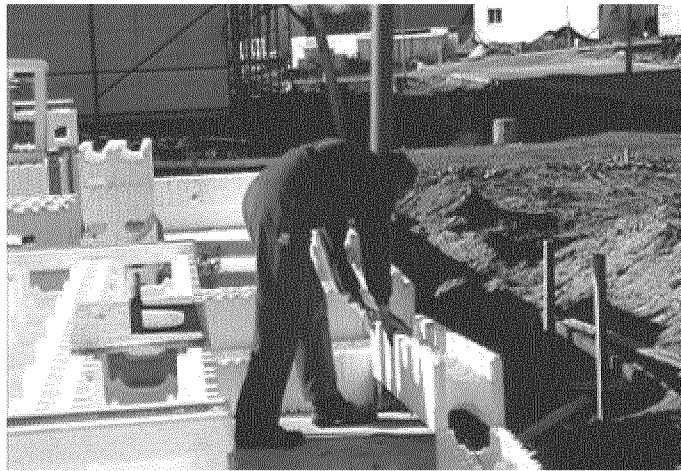
Рисунок 3 – Розкладання пінополістирольних блоків
