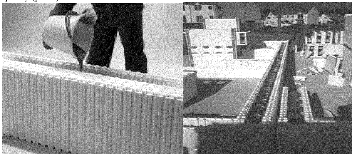
Рисунок 2 –Заливання бетону
