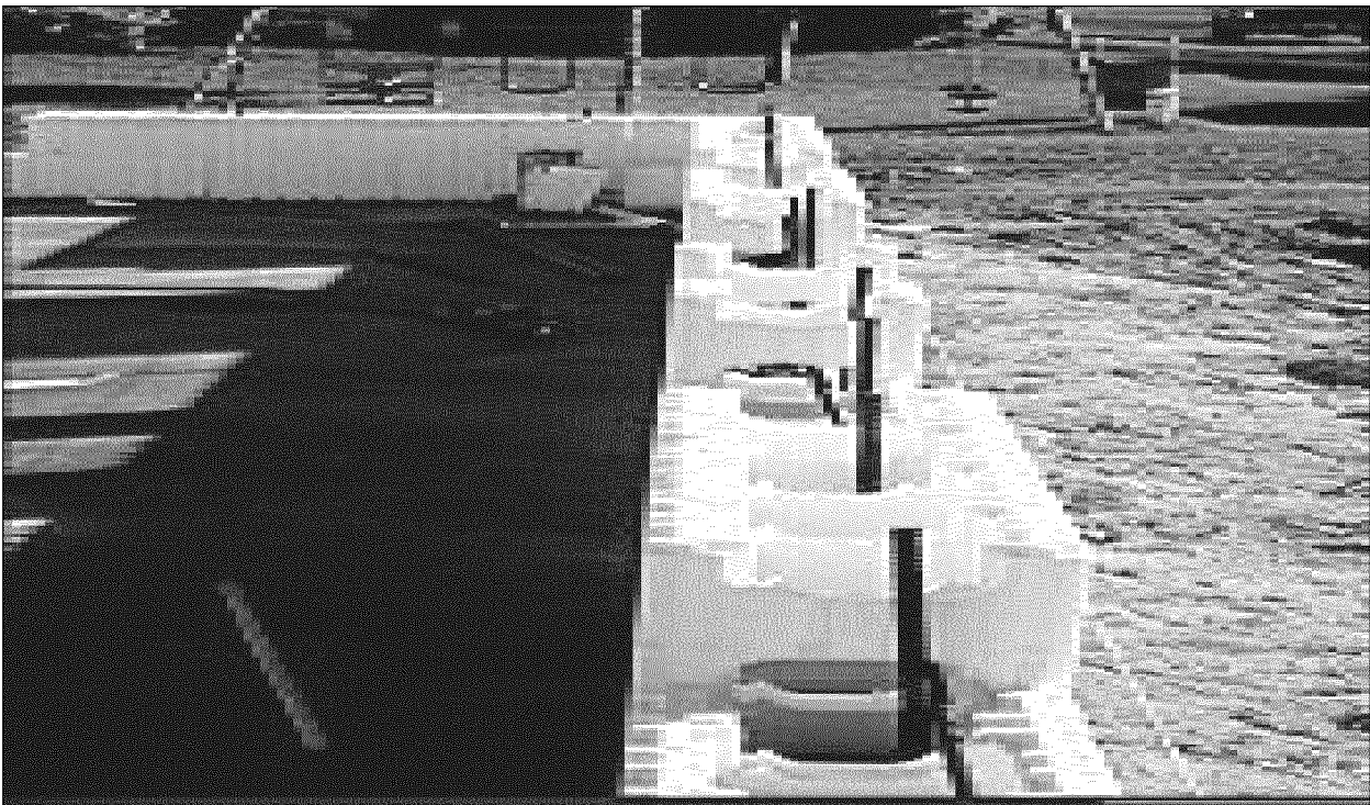
Рисунок 4 – Закладання арматури
