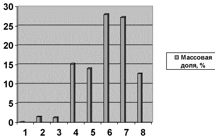
Рисунок 2 – Гистограмма распределения массовой доли частиц различной фракции
