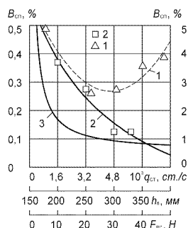
Рисунок – Зміна відходу стебел в плутанину B_{от} (ліва шкала) залежно від секундної їх подачі q_{ст} (1) в комбайн і висоти брання h_b (2) та впливу зусилля висмикування стебла F_{вс} (3) із затискного конвеєра на відхід стебел в плутанину B_{от} (права шкала)
