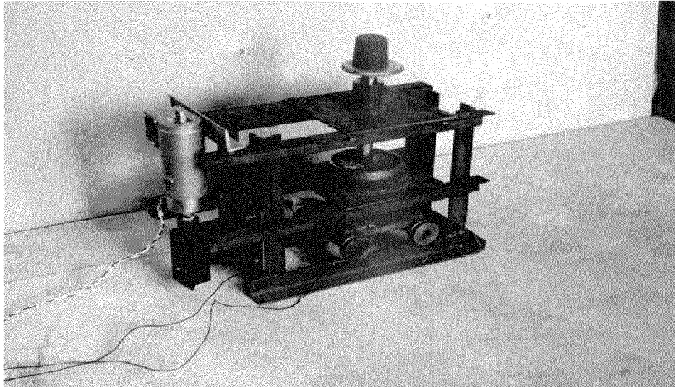
Рисунок 2 – Трибометр
