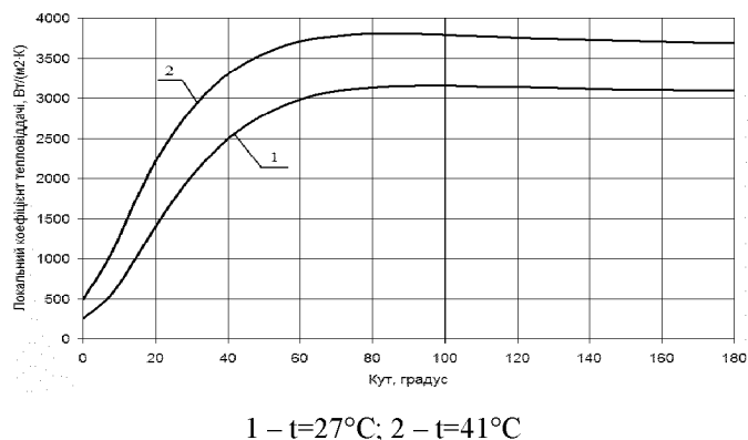
Рисунок 7 – Вплив температури на \alpha=f(\varphi) по периметру поперечного перерізу горизонтальної труби при q_{\text{зад}}=q_{\text{к}}=0 , q_{\text{роб}}=10160 \text{ Вт/м}^2
