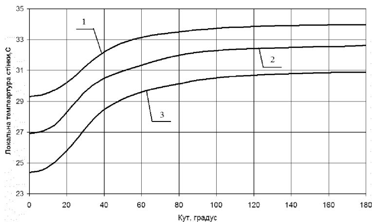
Рисунок 3 – Вплив густини теплового потоку на розподіл температури по периметру поперечного перерізу горизонтальної труби при температурі конденсації 40^\circ\text{C} та q_k=0 , q_{зад}=1100 \text{ Вт}
