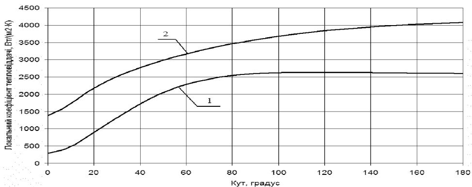
Рисунок 6 – Вплив швидкості пари на залежність \alpha=f(\varphi) по периметру горизонтальної труби при температурі конденсації 40^\circ\text{C} та q_{\text{зад}}=900 \text{ Вт} , q_{\text{роб}}=12800 \text{ Вт/м}^2
