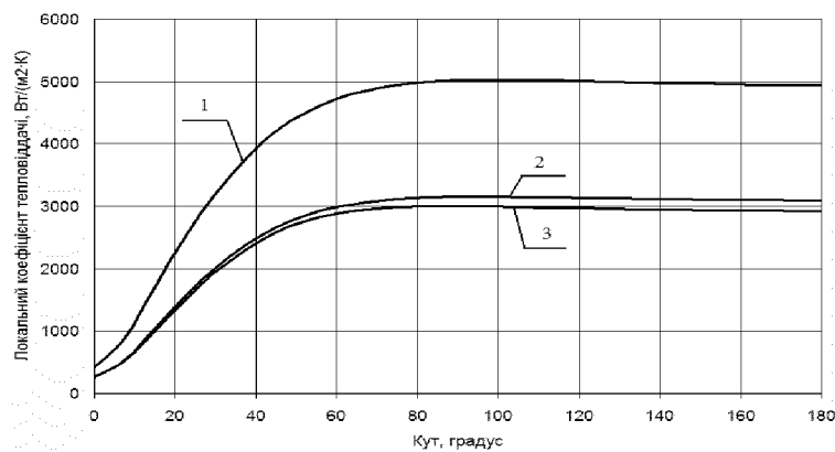
Рисунок 2 – Вплив густини теплового потоку на розподіл коефіцієнтів тепловіддачі по периметру поперечного перерізу горизонтальної труби при температурі конденсації 27^\circ\text{C} та q_{\text{зад}}=q_{\text{к}}=0
