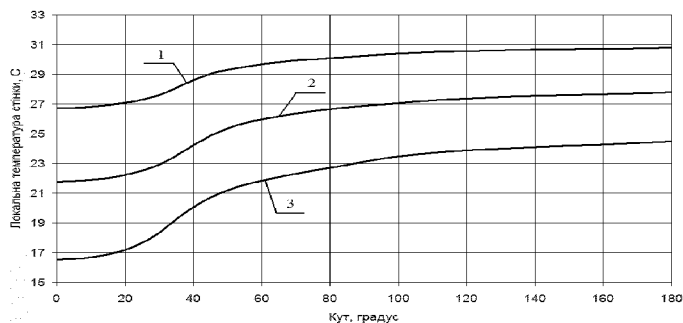
Рисунок 8 – Вплив густини теплового потоку на розподіл температури по периметру поперечного перерізу горизонтальної труби при температурі конденсації 37^\circ\text{C} та q_{\text{к}}=0
