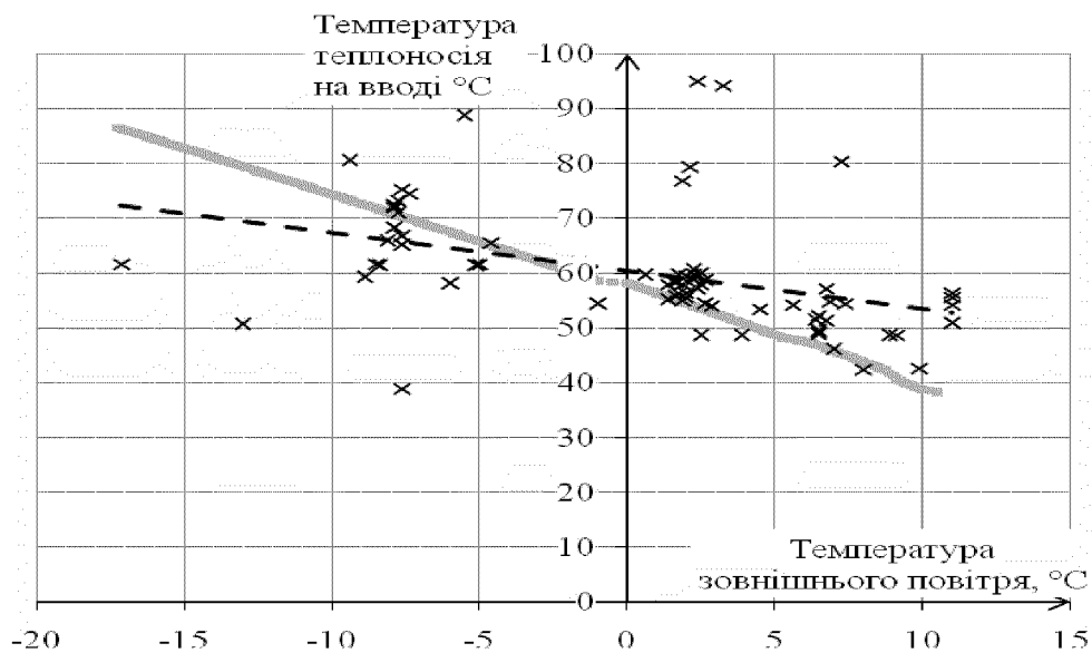
Рисунок 3 - Розкид температур теплоносія (точки ×), апроксимований прямою 1, відносно нормативних значень на ввіді (крива 2)
