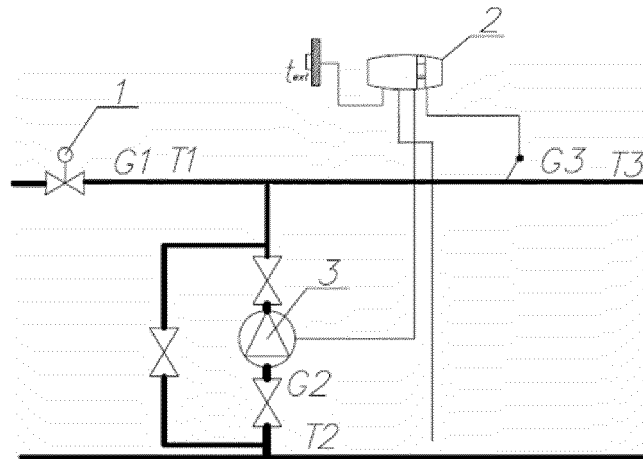
Рисунок 6 - Схема елеваторного вузлу системи опалювання з відцентровим насосом на перемичці 1 - регулятор перепаду тиску; 2 - контролер; 3 - відцентровий насос
