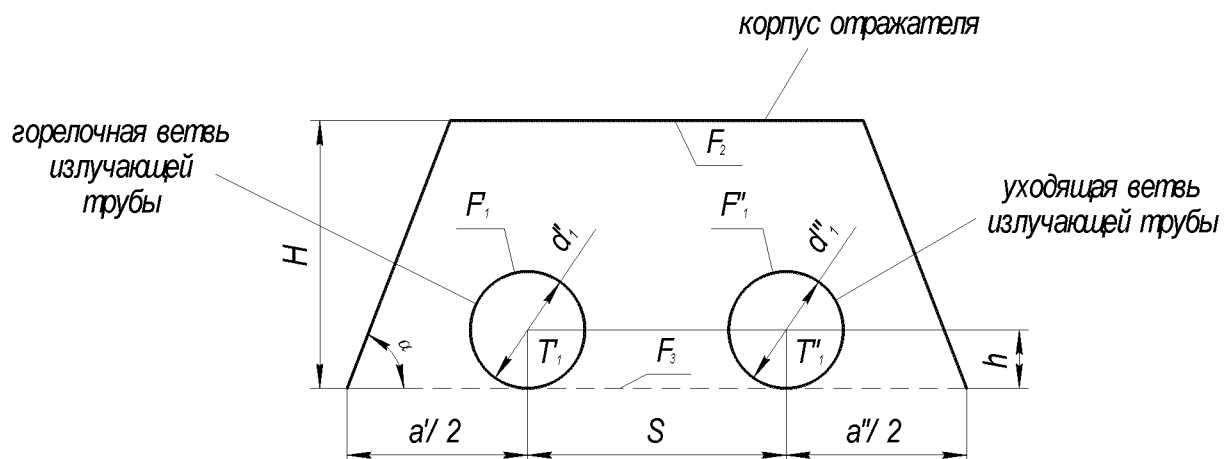
Рисунок 2 – Основные элементы U-образного излучателя (внутренний контур)
