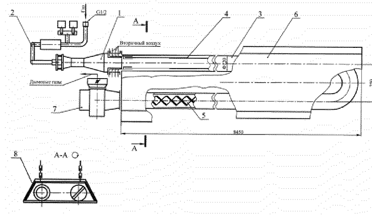
Рисунок 1 - Конструктивная схема U-образного излучателя
