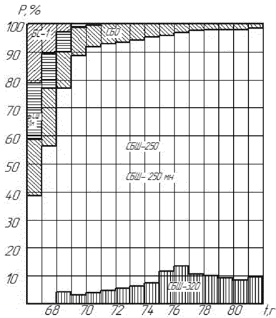
Рисунок 1 – Графіки зміни електричного навантаження при використанні бурових станків на кар'єрах Кривбасу
