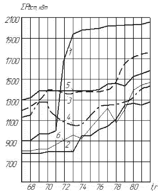
Рисунок 2 – Графіки зміни електричного навантаження при використанні екскаваторів на кар'єрах Кривбасу
