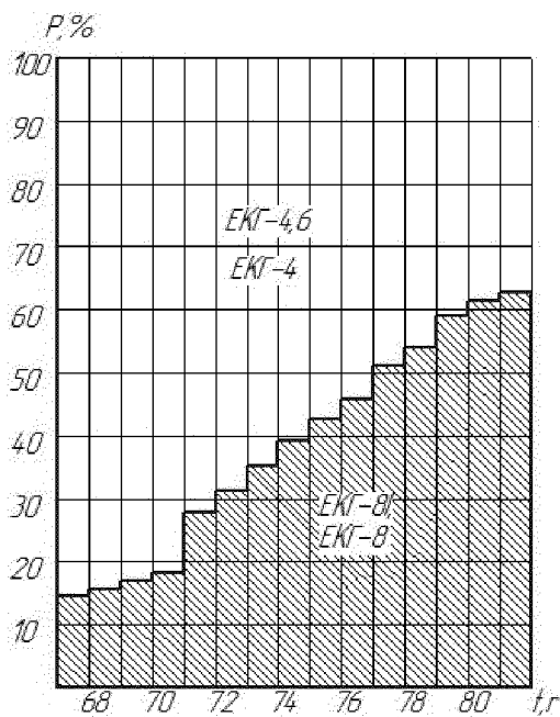
Рисунок 2 – Графіки зміни електричного навантаження при використанні екскаваторів на кар'єрах Кривбасу
