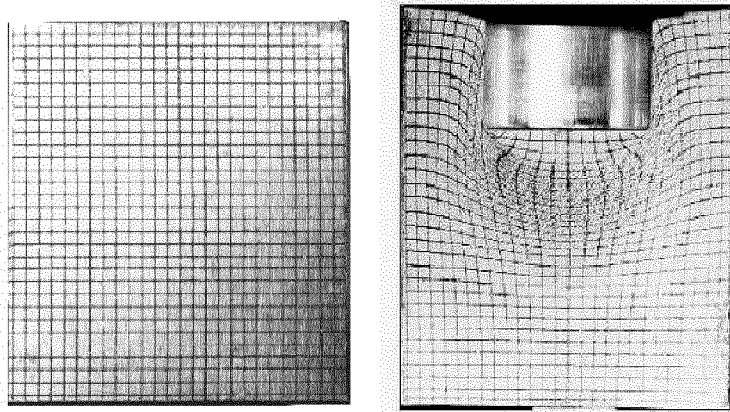
Рисунок 2 – Зміни координатної сітки на недеформованому (ліворуч) та деформованому (праворуч) зразку
