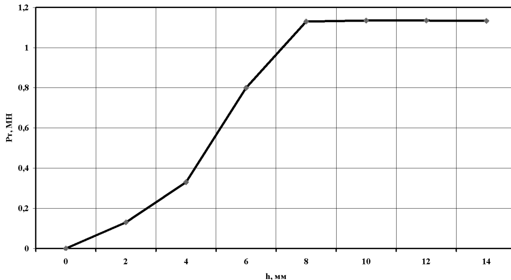
Рисунок 7 – Експериментальний графік технологічного зусилля видавлювання
