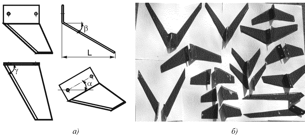
а) геометричні параметри плоскоріжучого ножа; б) набір ножів для експериментальних досліджень
