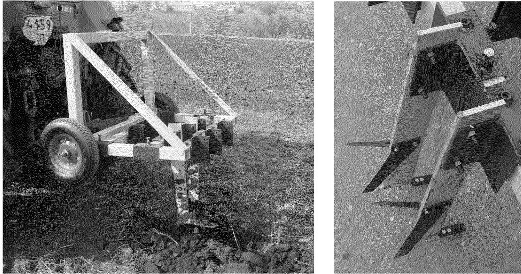
Рисунок 4 - Експериментальний адаптивний розпушувач ґрунту та його робочі органи
