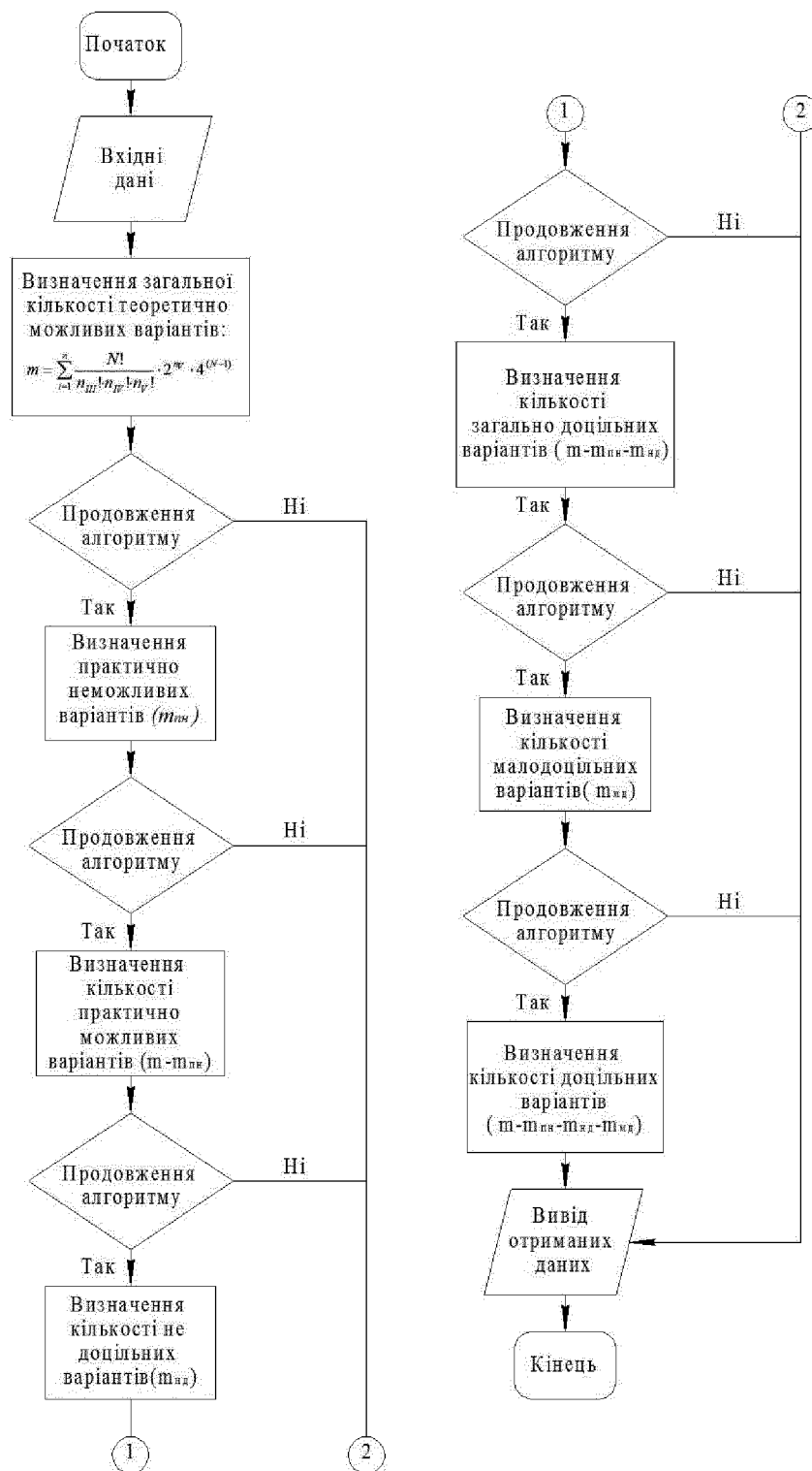
Рисунок 1 – Блок-схема визначення доцільних варіантів кінематичних схем промислових роботів
